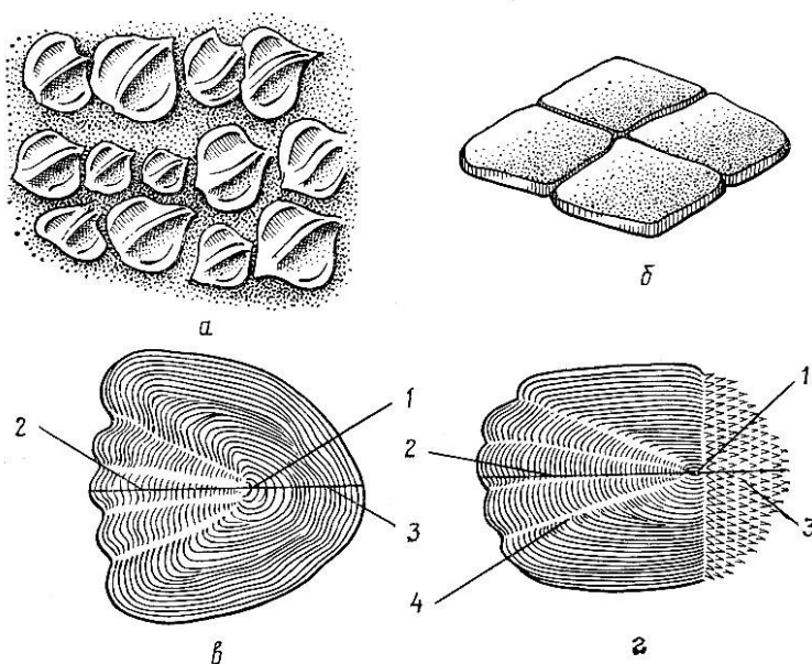
Рисунок 22 – Типы чешуи:
