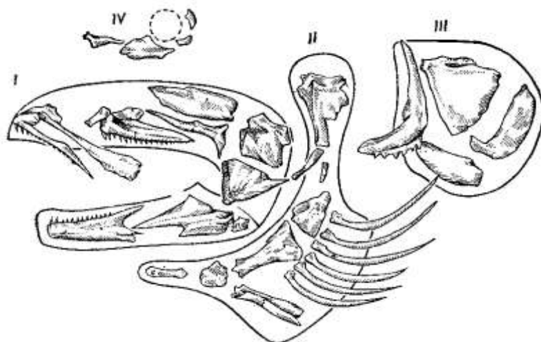
Рисунок 54 – Схема расположения костей висцерального скелета головы судака:
