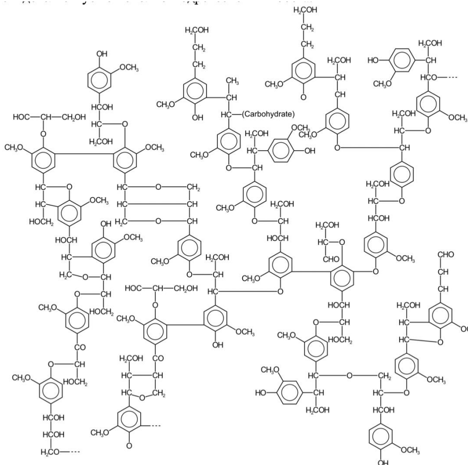
Рис. 1. Структура лигнина
