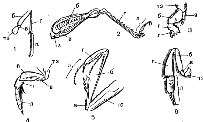
Рис. 34. Строение и типы ног насекомых: 1 — бегательная (жулици); тз — тазик, в — вертлуг, б — бедро, г — голень, л — лапка; 2 — прыгательная (сараңчи); 3 — копательная (медведки); 4 — плавательная (плавунца); 5 — хватательная (богомол); 6 — собирательная (пчелы).
